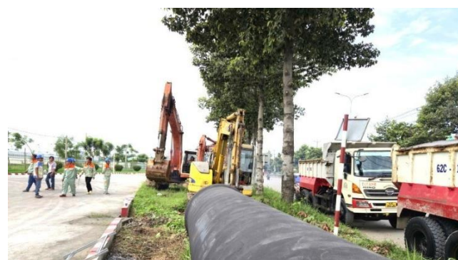
Ống truyền tải cấp nước có đường kính D1200 và trang thiết bị đã tập kết để thi công.
